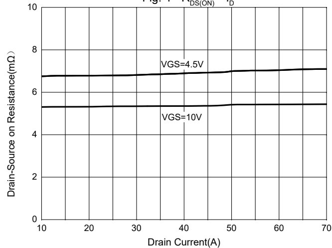
Fig. 4 - R_{DS(ON)} - I_D
