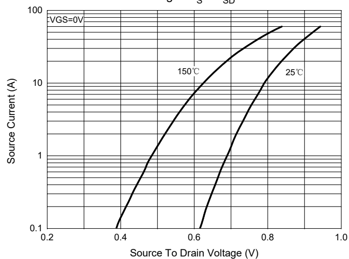
Fig.9 - I_S - V_{SD}
