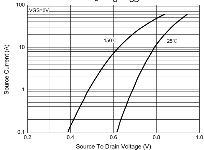
Fig.9 - I_S - V_{SD}
