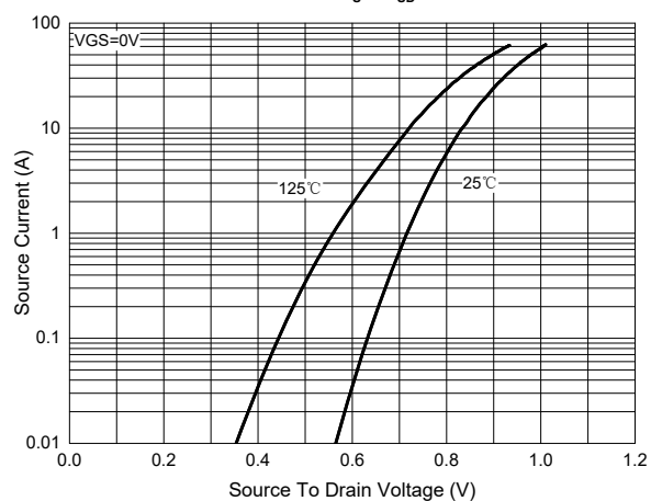
Fig.9 - I_S - V_{SD}
