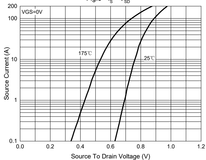
Fig.9 - I_S - V_{SD}
