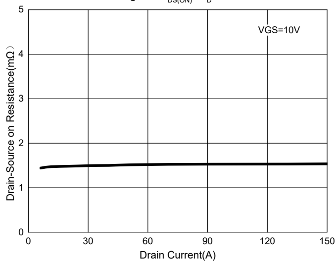
Fig. 4 - R_{DS(ON)} - I_D
