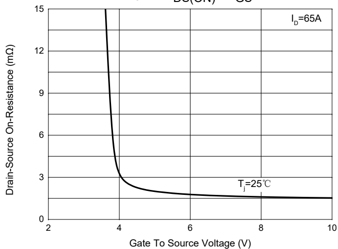
Fig. 3 - R_{DS(ON)} - V_{GS}
