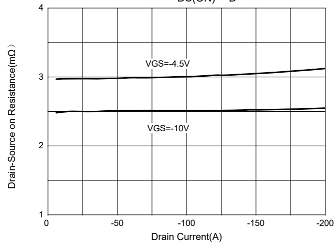
Fig. 4 - R_{DS(ON)}-I_D
