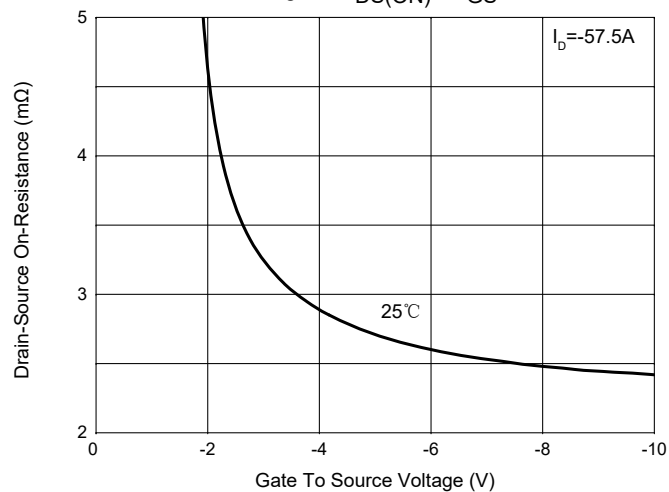
Fig. 3 - R_{DS(ON)}-V_{GS}
