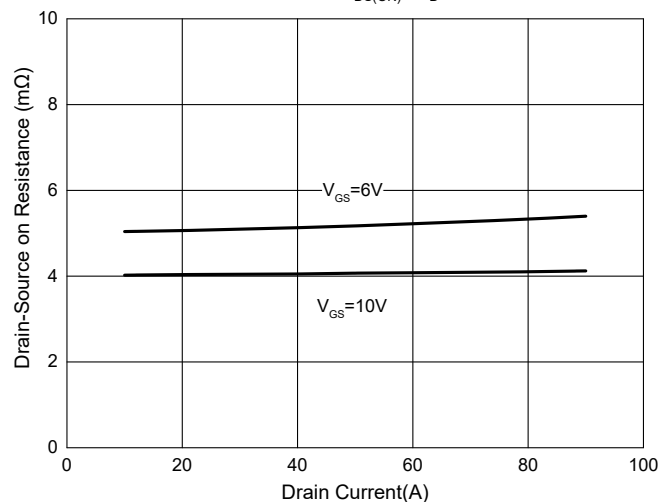
Fig. 7 - R_{DS(ON)} - I_D
