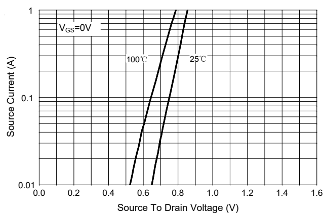
Fig.9 - I_S - V_{SD}
