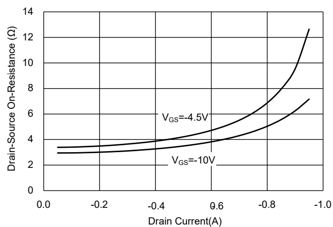
Fig.4 RDS(ON)-ID
