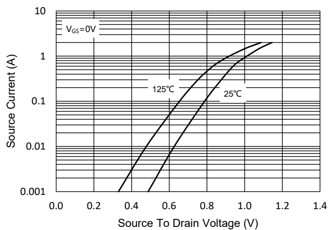
Fig.9 - I_S - V_{SD}
