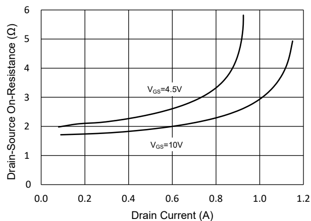
Fig.4 - R_{DS(ON)} - I_D
