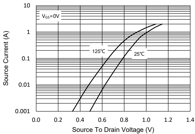
Fig.9 - I_S - V_{SD}
