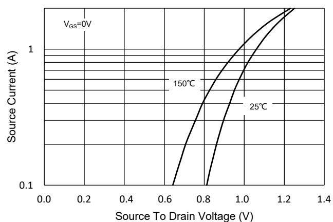
Fig.9 - I_S - V_{SD}
