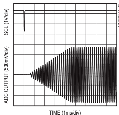
SOFT-START ADC
