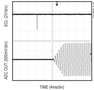
ADC SOFT-START
