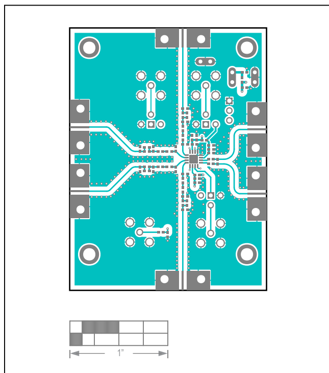
Top
