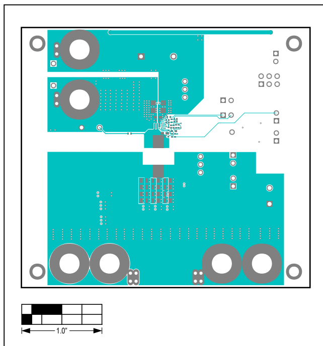
MAX38802 EV Kit—Top
