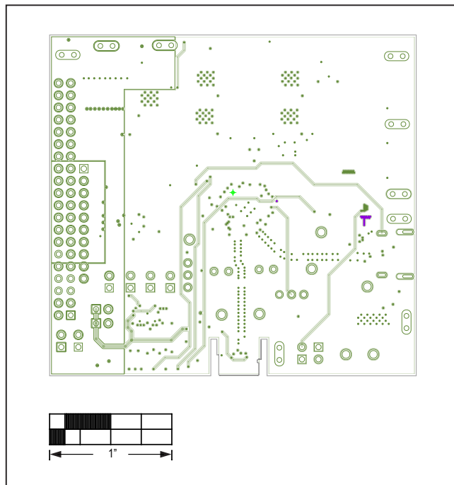
MAX25430A EV Kit PCB Layout - Layer 6
