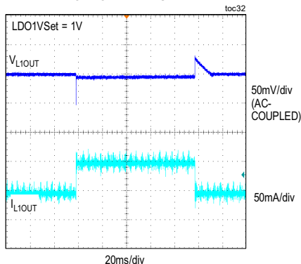
LDO1 LOAD TRANSIENT
