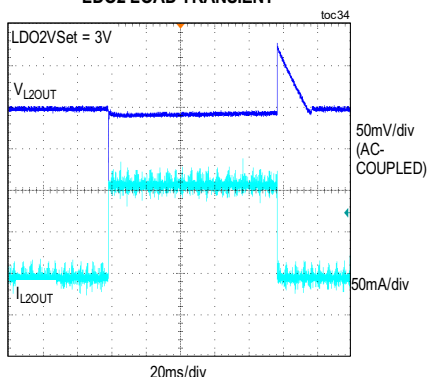
LDO2 LOAD TRANSIENT
