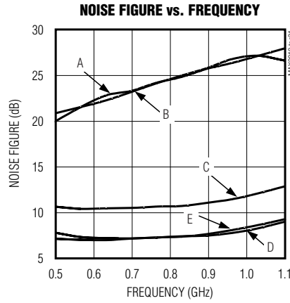
A = V_{GCS} = 0V , V_{GFS} = 0V D = V_{GCS} = 5V , V_{GFS} = 0V B = V_{GCS} = 0V , V_{GFS} = 5V E = V_{GCS} = 5V , V_{GFS} = 5V C = V_{GCS} = 1.5V , V_{GFS} = 5V
