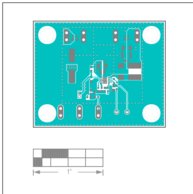
MAX17783C EV Kit—Top Layer
