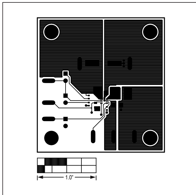
MAX15062AEVKIT# EV Kit—Top Layer
