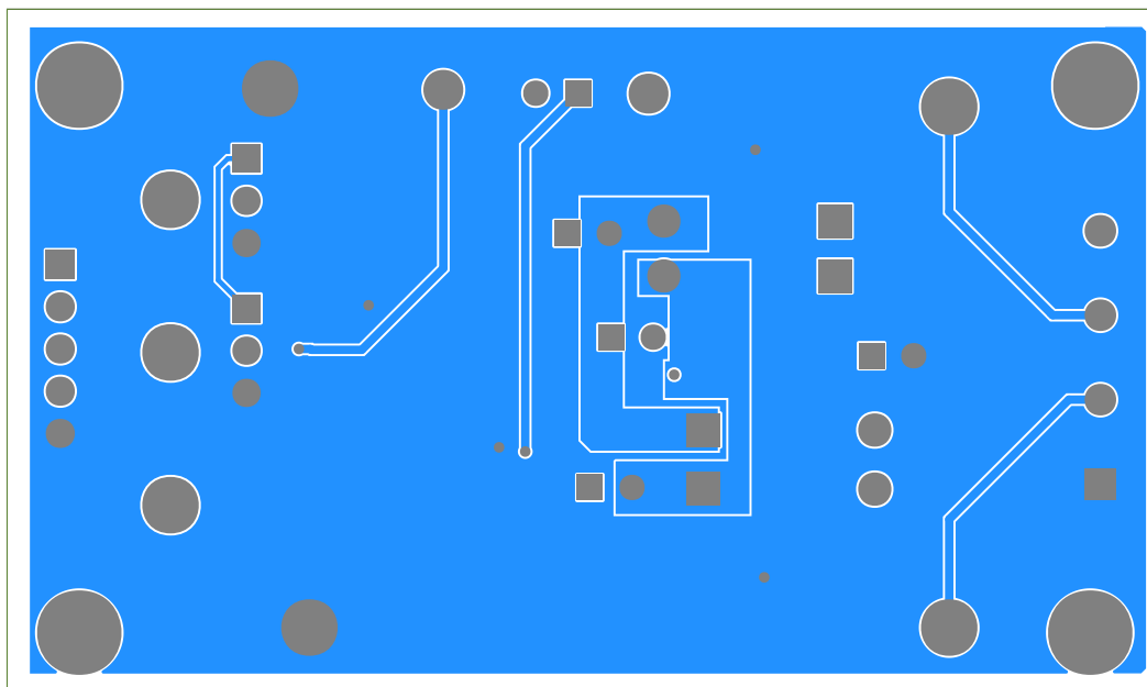
MAX14883E EV Kit—Bottom Layer
