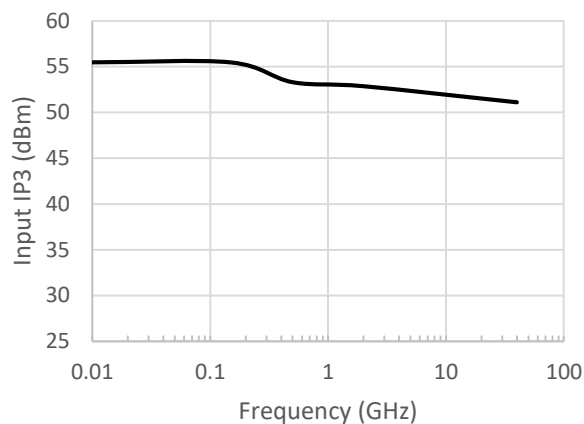
Input IP3 13
