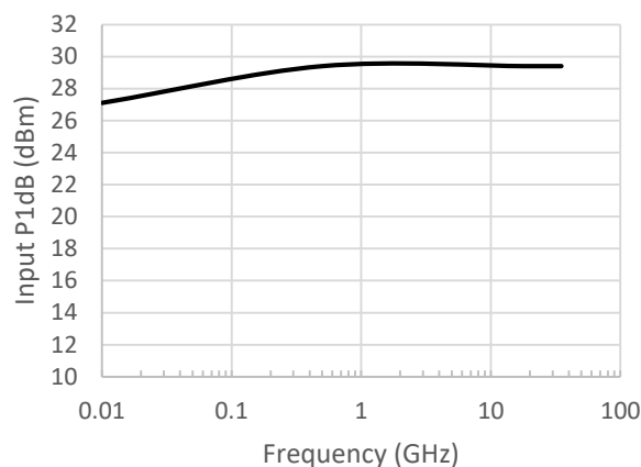
Input P1dB
