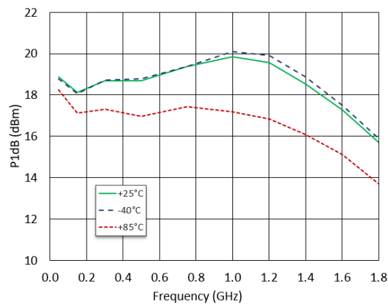
P1dB
