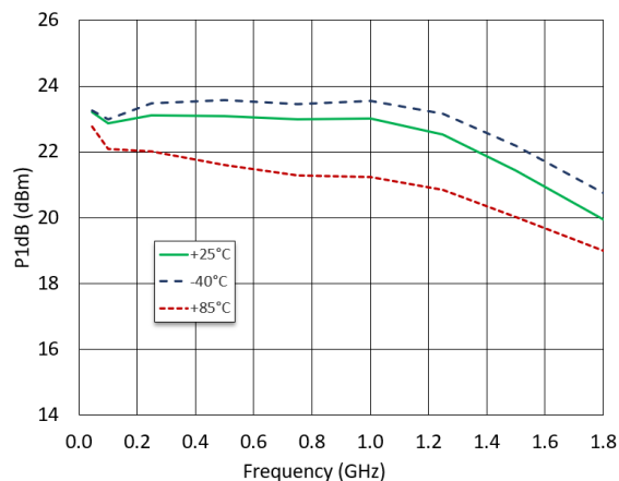
P1dB
