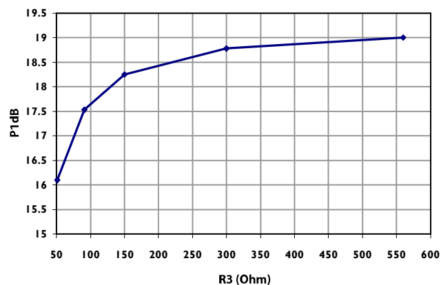
P1dB
