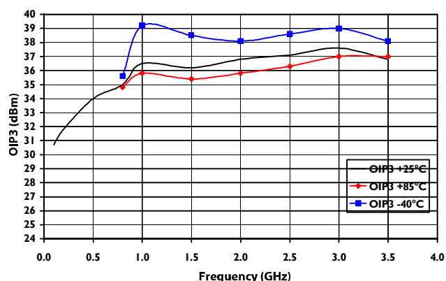
OIP3
