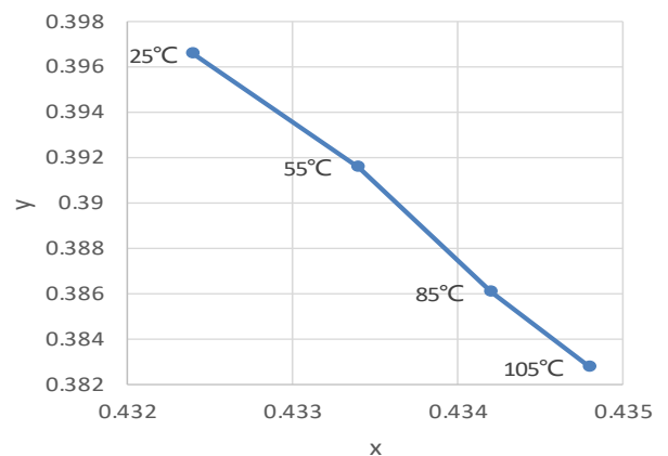
SOLDERING TEMP. VS. CIE X, Y SHIFT
