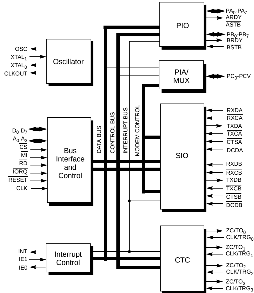
Figure 1. KIO Block Diagram
