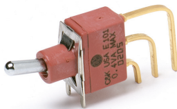
E101MD1AV2BE Vertical Actuation SPDT
