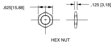
HEX NUT
