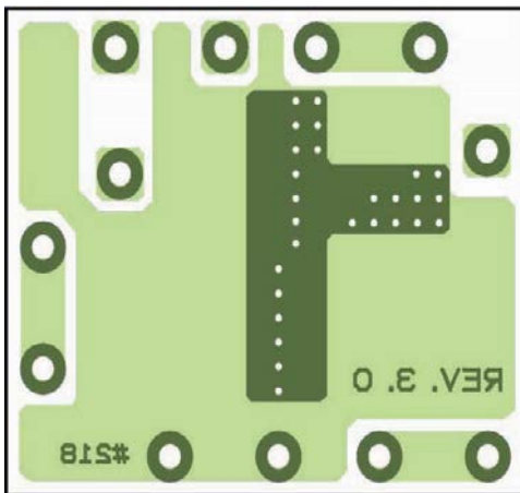
SOT-25 (Back)
