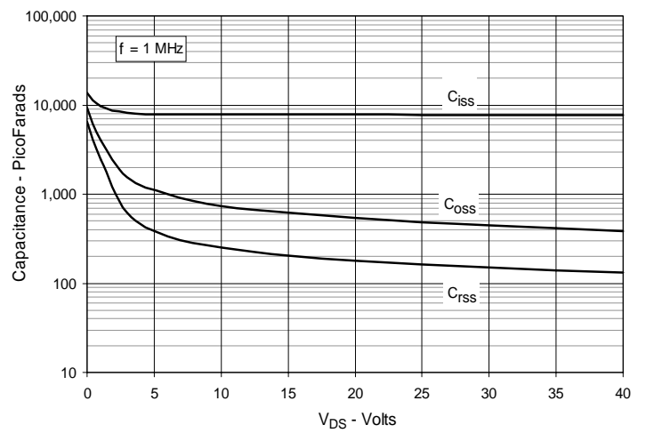
Fig. 10. Capacitance
