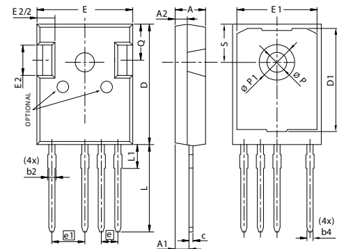
L014d TO-247-4L g
