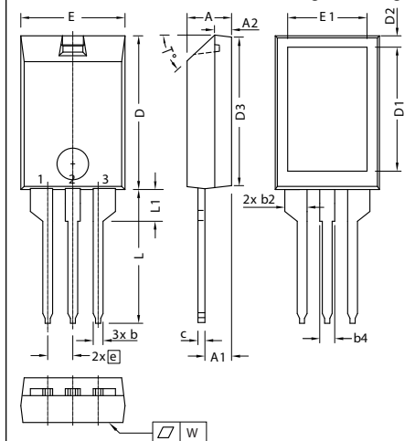
X010a ISOPLUS220™ AB
