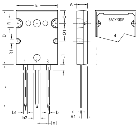
X021a PLUS264™
