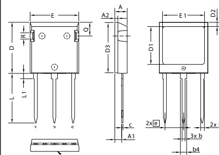
X024b ISOPLUS i4-PAC™
