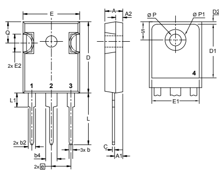
X014a TO-247 AD
