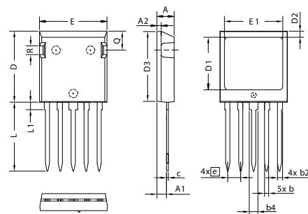
X024a ISOPLUS i4-PAC™
