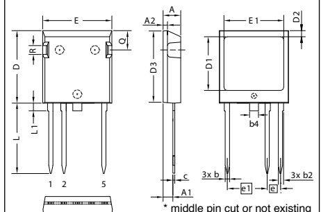
X024c ISOPLUS i4-PAC™
