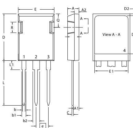
X015a PLUS247™
