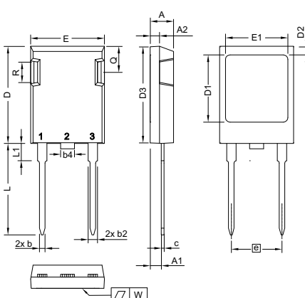
X016b ISOPLUS247™
