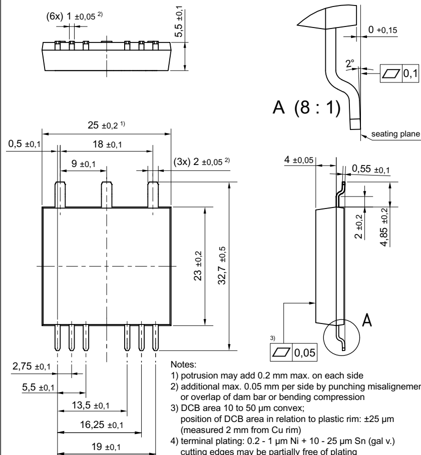
X030a SMPD-B
