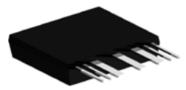
X030b SMPD-B
