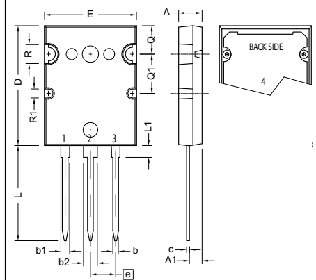
X021a PLUS264™
