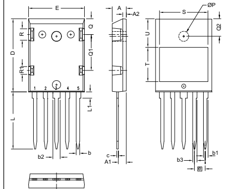
X023 ISO264™
