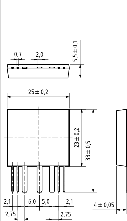
X030b SMPD-B
