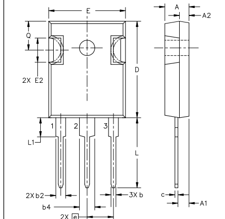
X016c ISO247™
