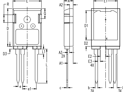
X015c PLUS247™
