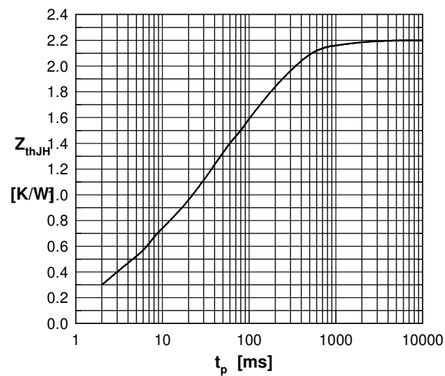
Fig. 8 Typ. transient thermal impedance
