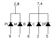
D.LTS-6x95
