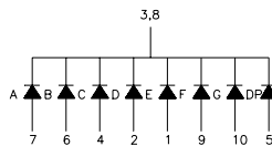
B.LTS-6x80
