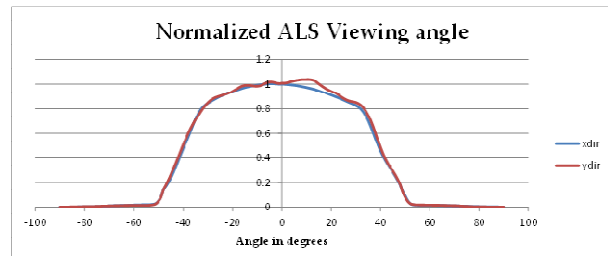
Figure 4.2 ALS Sensitivity vs. Angular of Incidence
