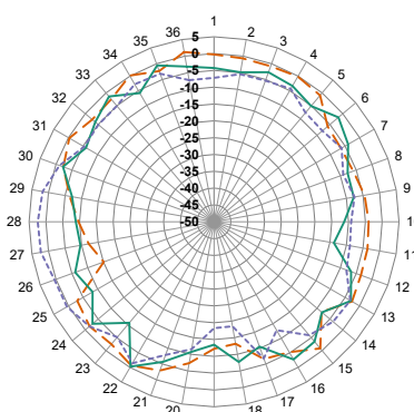
YZ-Plane Gain
