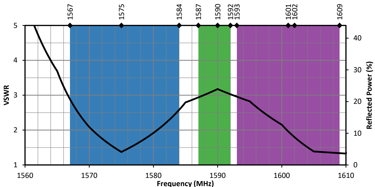
Figure 1. GNSSCP-TH18L1 VSWR
