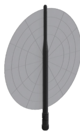
YZ-Plane Gain
