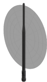
XZ-Plane Gain
