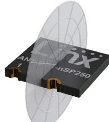
YZ-Plane Gain
