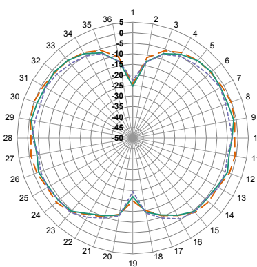
XZ-Plane Gain
