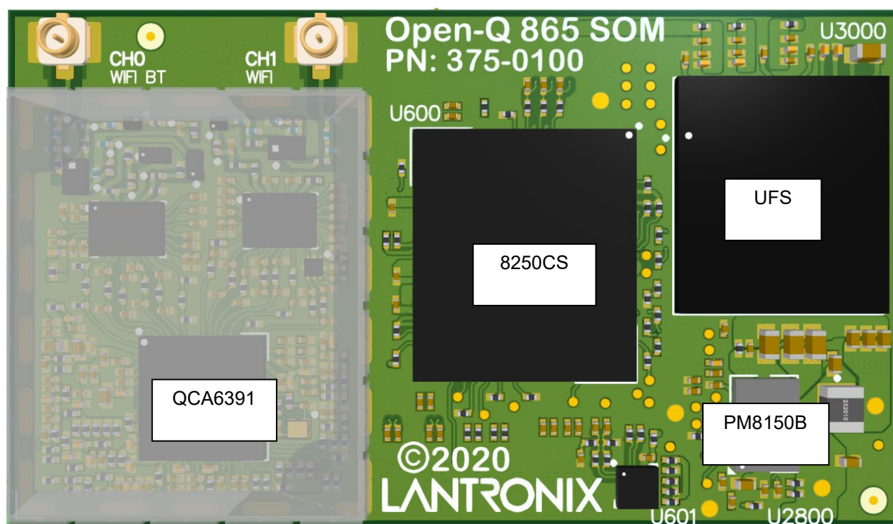
Figure 2. Open-Q 8250CS SOM Top View
