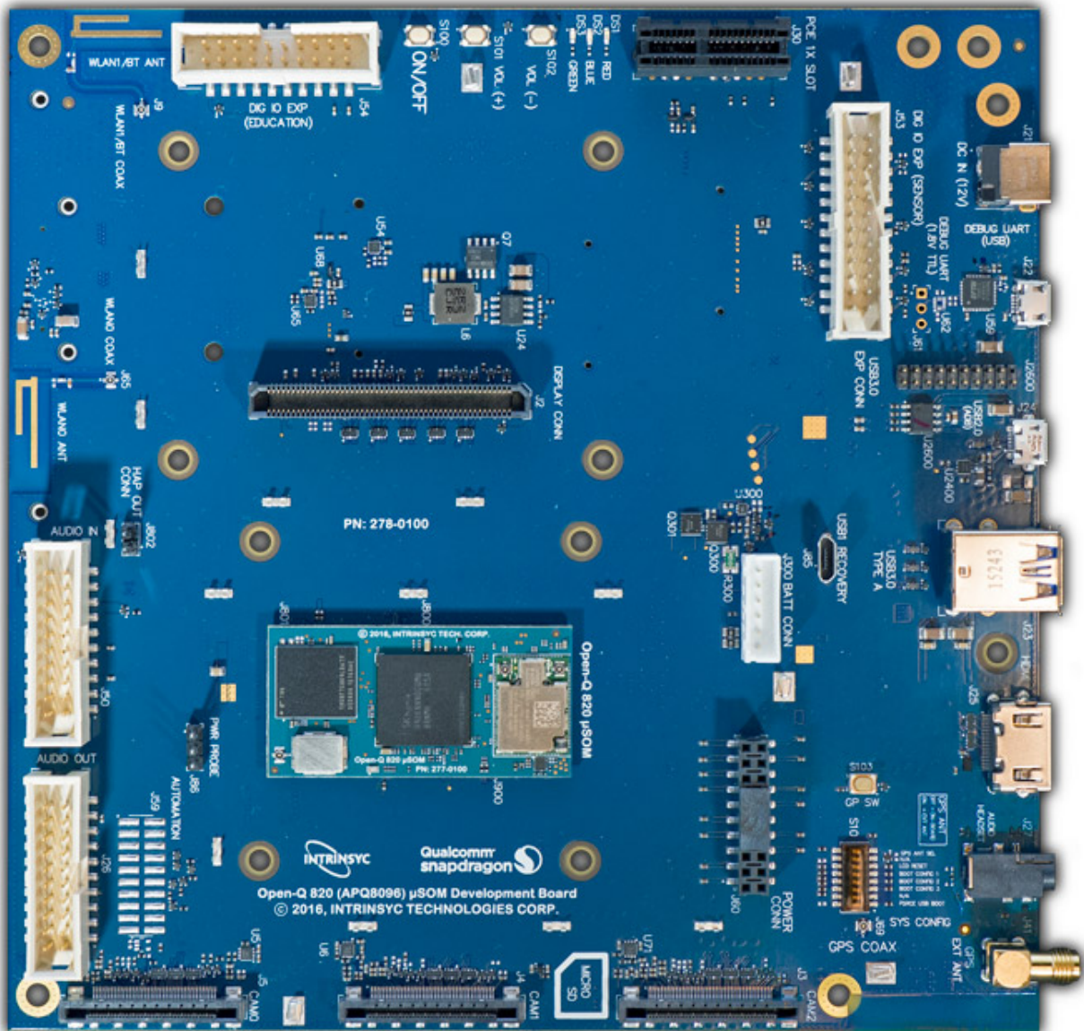
Figure 1 Assembled Open-Q 820 / 820Pro \mu SOM Development Kit
