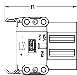
Stecker-Draufsicht
