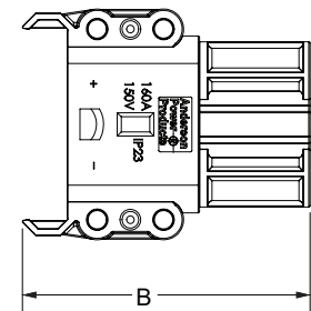
Gehäuse-Draufsicht
