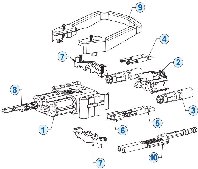
Steckerbuchse
