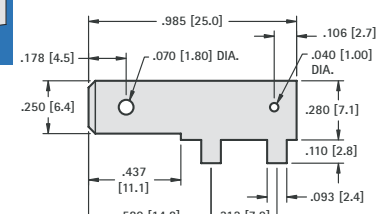
.250 (6.4) TAB
