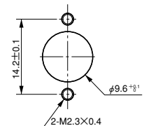
パネル取付穴寸法 (参考) PANEL MOUNTING HOLE PATTERNS (REF.)
