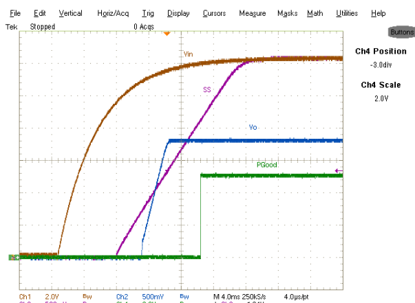
Fig. 18. Start up at 2A Load, Ch 1 : V_{in} , Ch 2 : V_o , Ch 3 : V_{ss} , Ch 4 : V_{PGGood}
