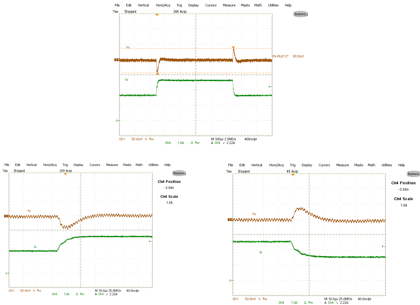
Fig. 23. Transient Response, 1A to 2A step 2.5A/µs Ch 1 : V_o , Ch 4 : I_o
