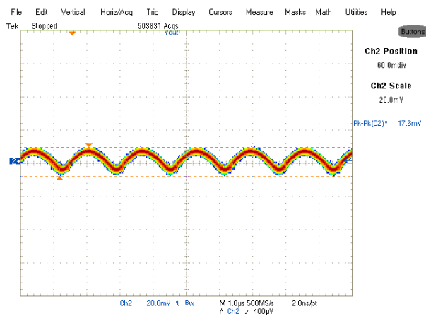
Fig. 20. Output Voltage Ripple, 2A load Ch 2 : V_o
