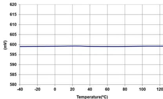
OVP_Vth
